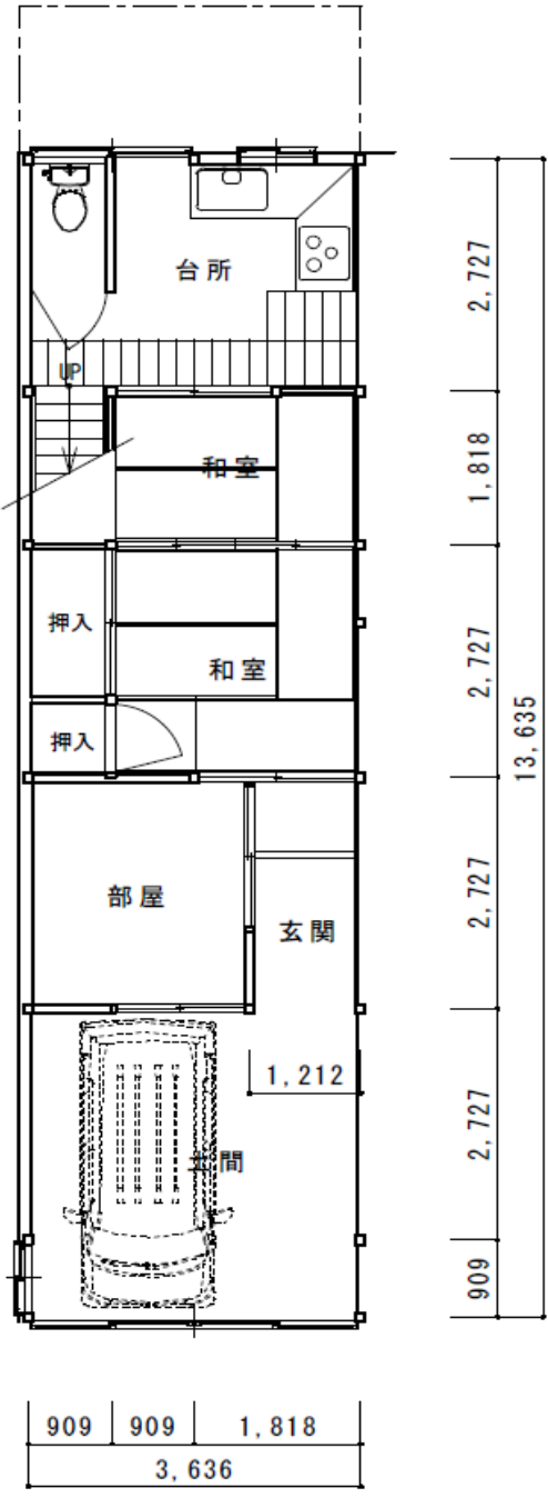
一階平面図
