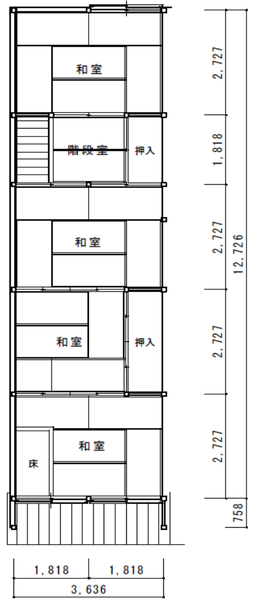
二階平面図
